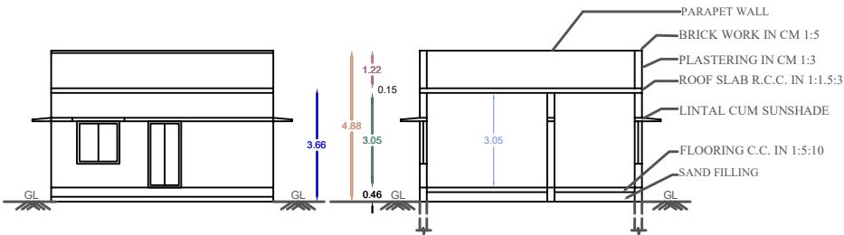
ELEVATION
