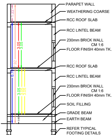
SECTION A-B
