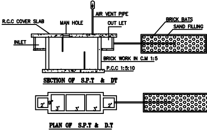
PLAN OF S.P.T & D.T
