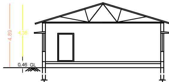
SECTION NO A-A
