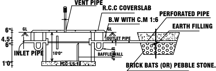
SECTION OF S.P.T & D.T
