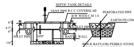
SECTION OF S.P.T & D.T
