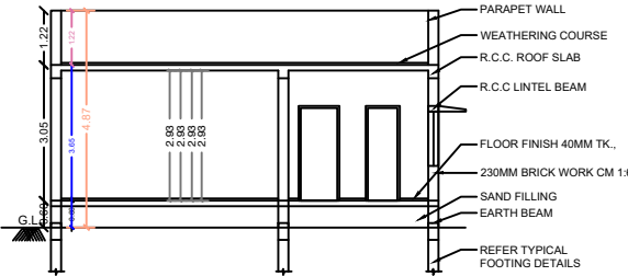
SECTION A-B
