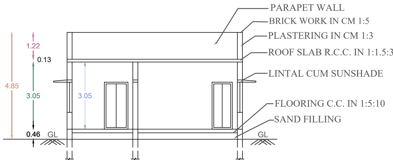
SECTION NO A-A
