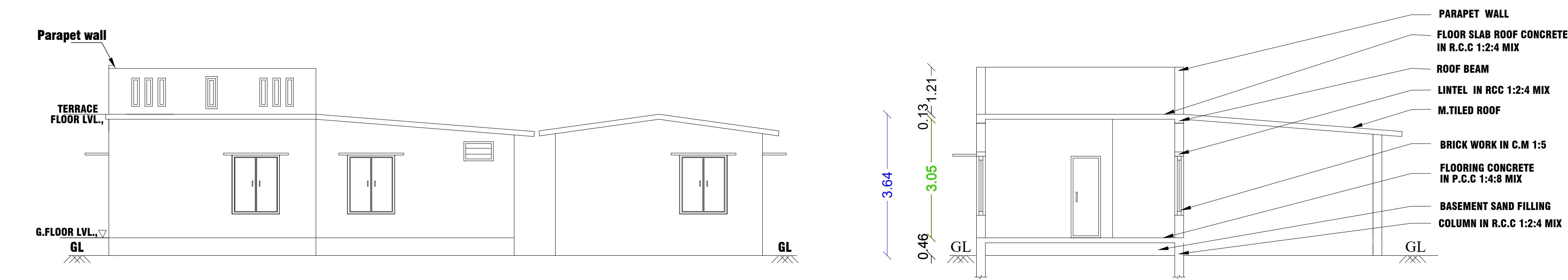
ELEVATION
