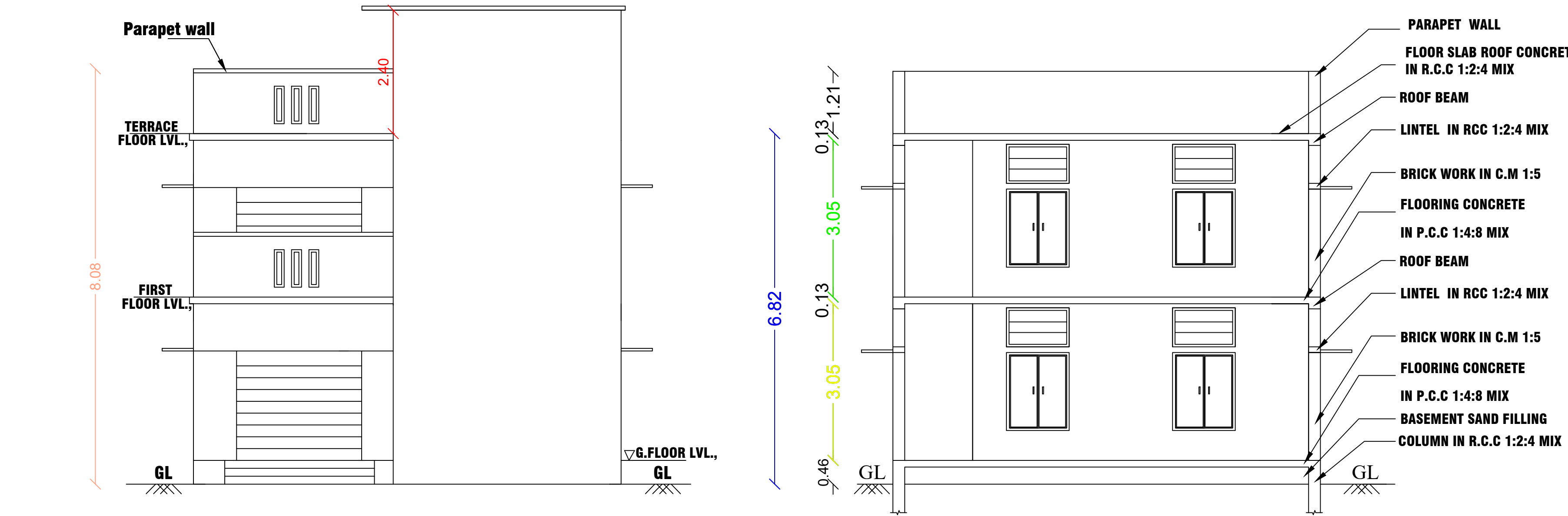
ELEVATION
