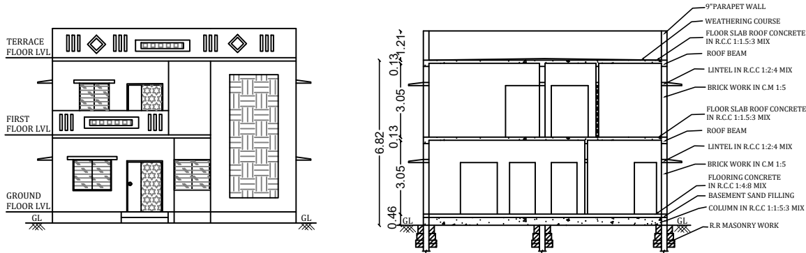
ELEVATION
