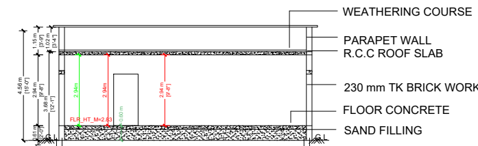
SECTION - AB
