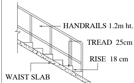
STAIRCASE DETAILS (N.T.S.)
