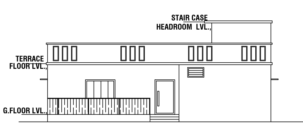
ELEVATION
