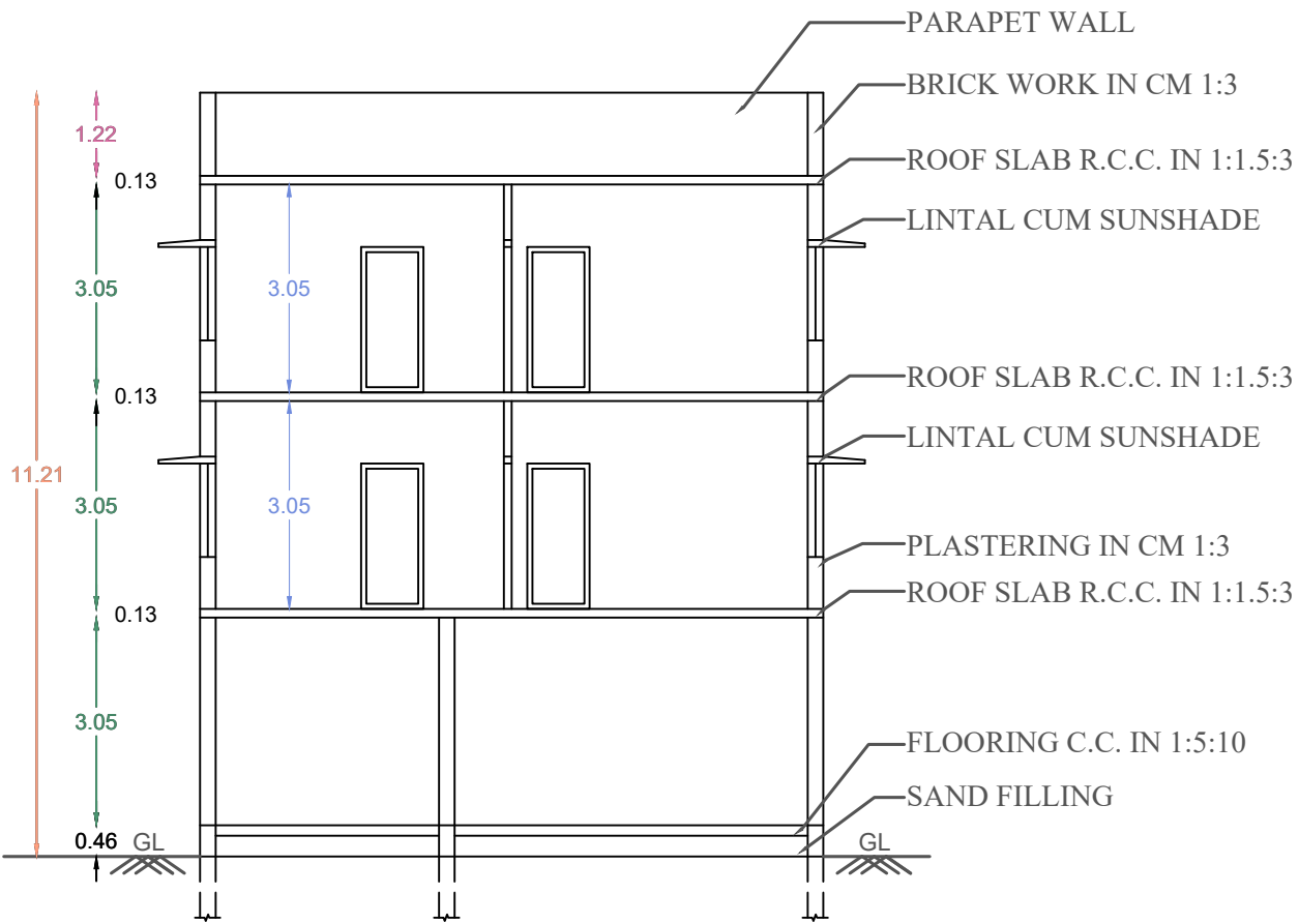
SECTION NO A-A
