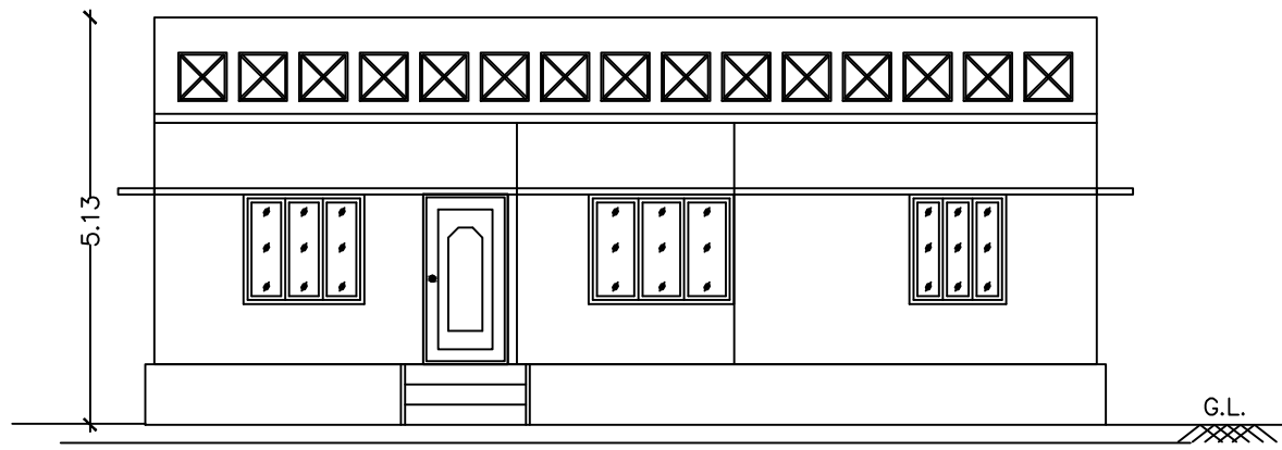
ELEVATION
