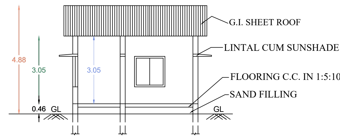
SECTION NO A-A
