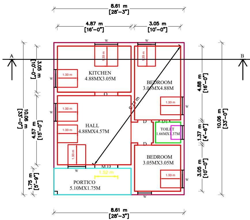
PLAN SCALE ( 1 : 100 )
