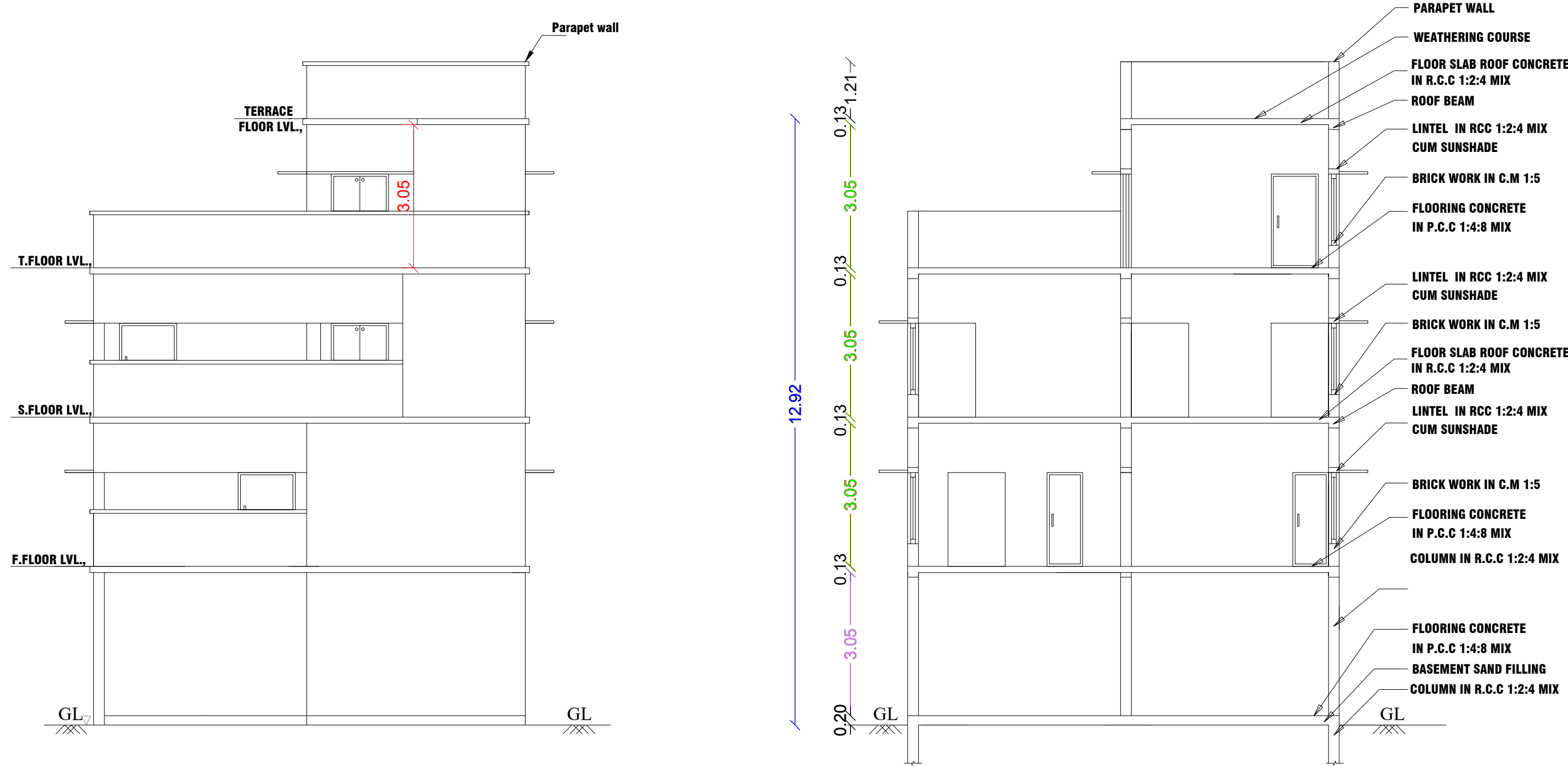
ELEVATION
