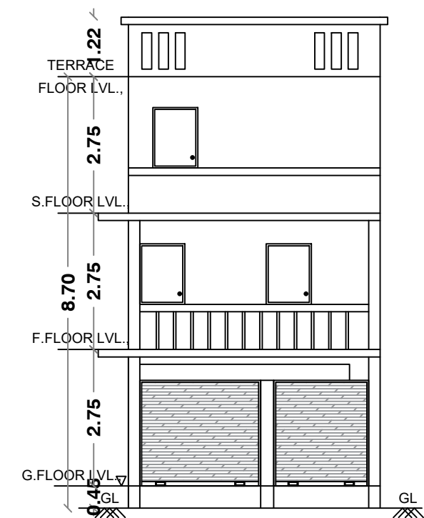
ELEVATION
