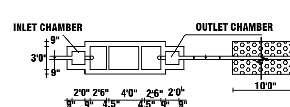
PLAN OF S.P.T & D.T
