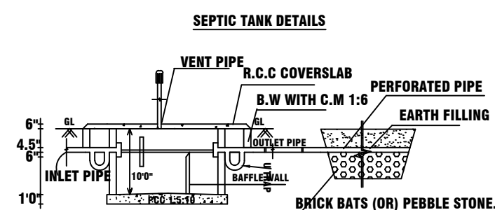
SECTION OF S.P.T & D.T
