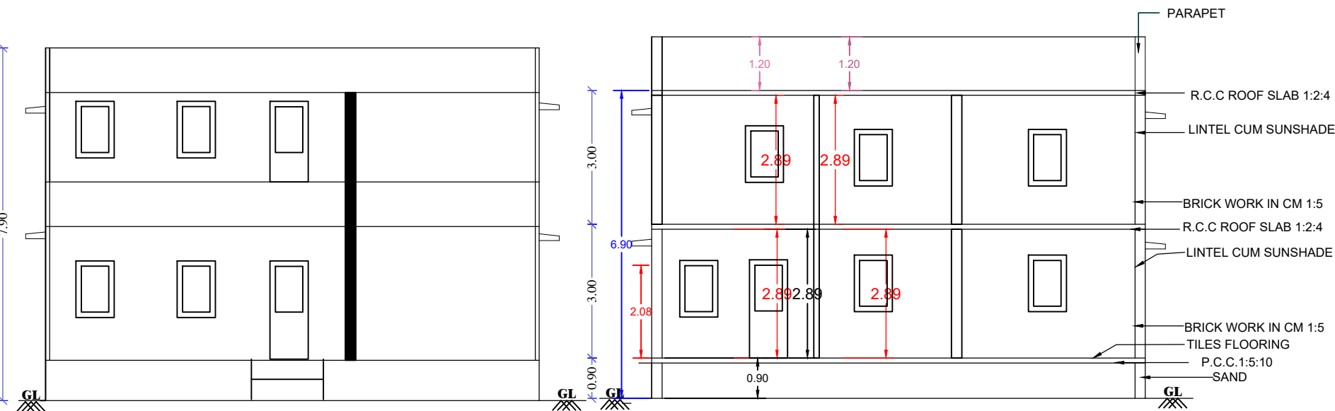
ELEVATION
