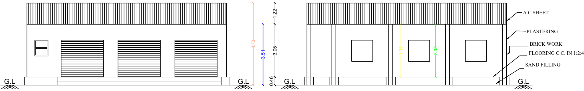
ELEVATION
