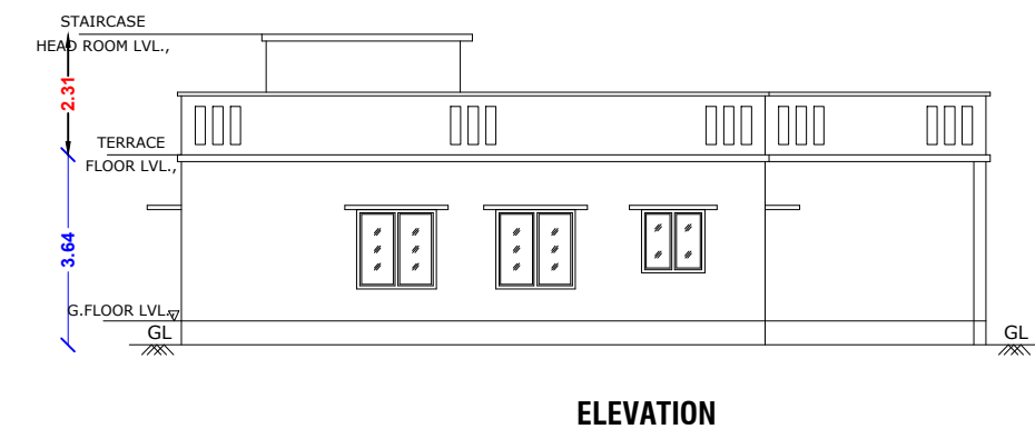
ELEVATION
