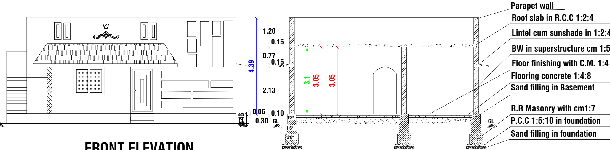
SECTION A-A
