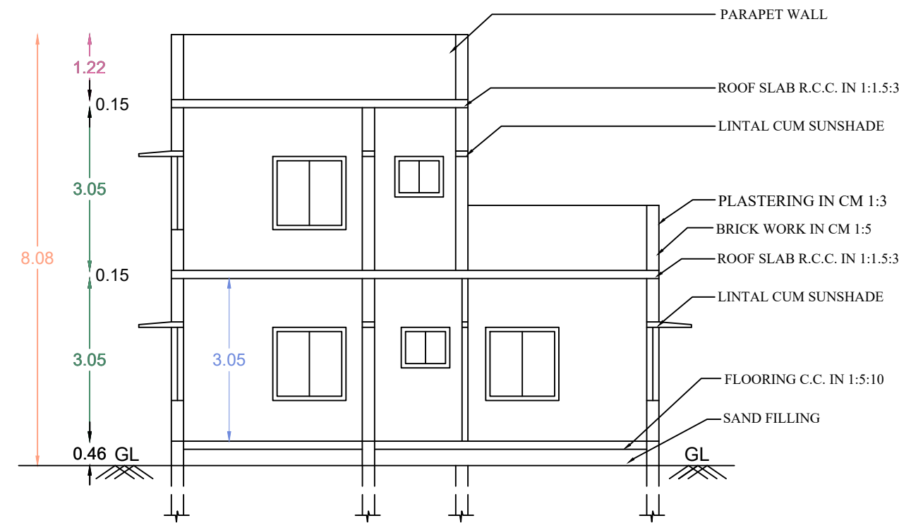
SECTION NO A-A
