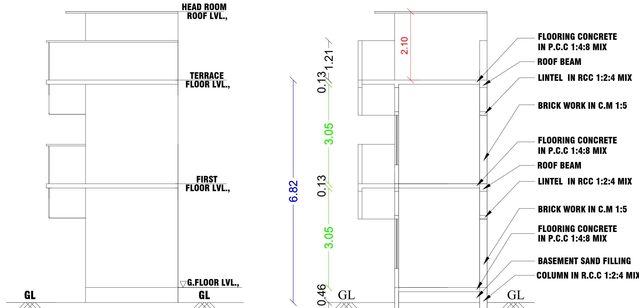
ELEVATION
