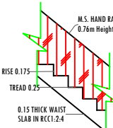
STAIRCASE DETAILS SCALE: 1:20
