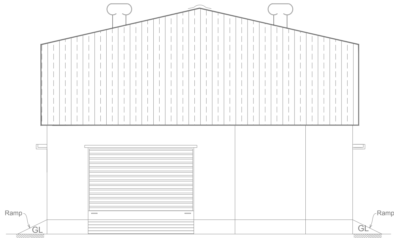
ELEVATION
