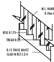
STAIRCASE DETAILS SCALE: 1:20
