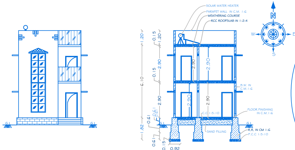
ELEVATION
