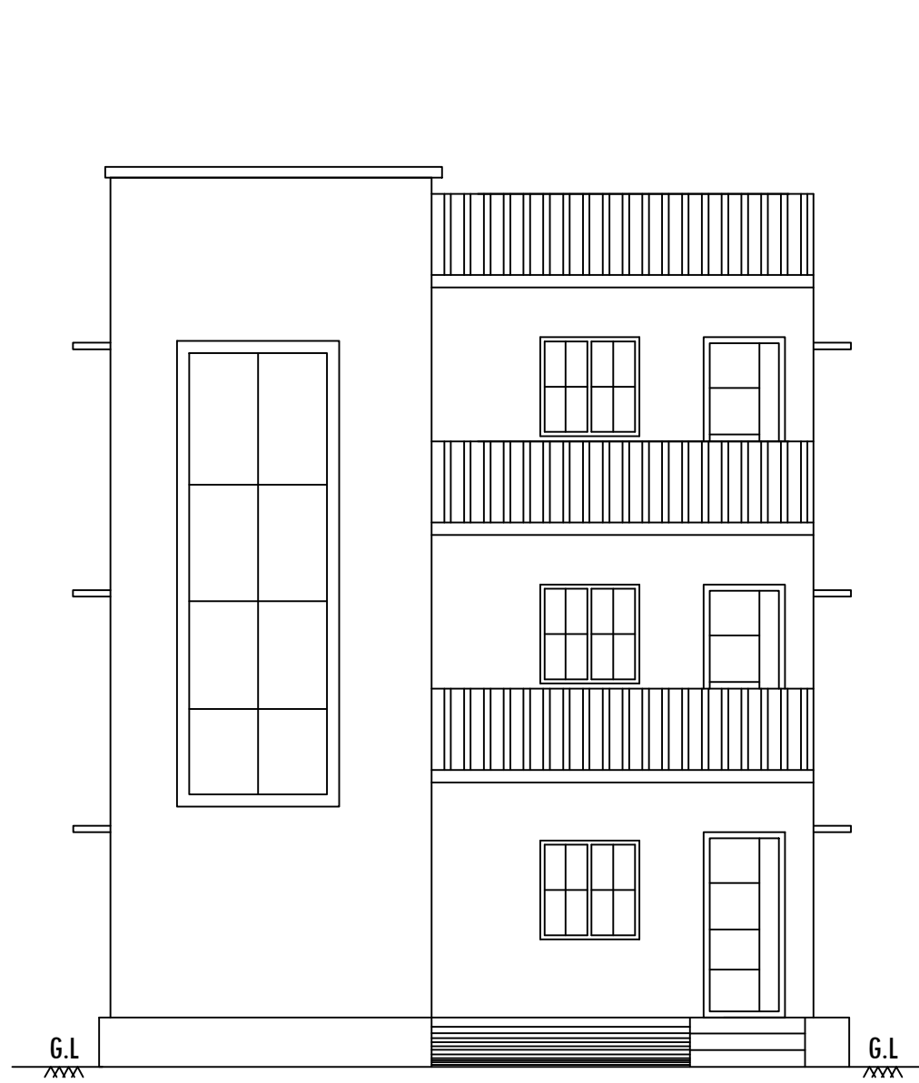
ELEVATION
