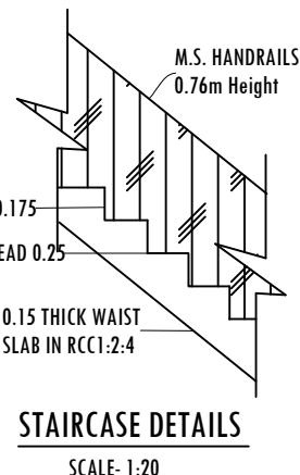
STAIRCASE DETAILS SCALE: 1:20
