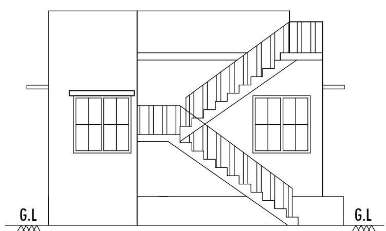
ELEVATION
