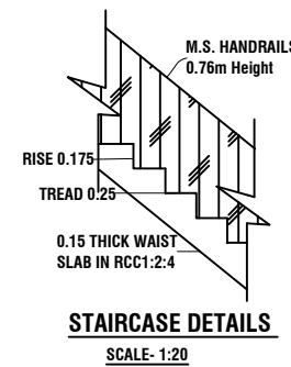
STAIRCASE DETAILS SCALE: 1:20
