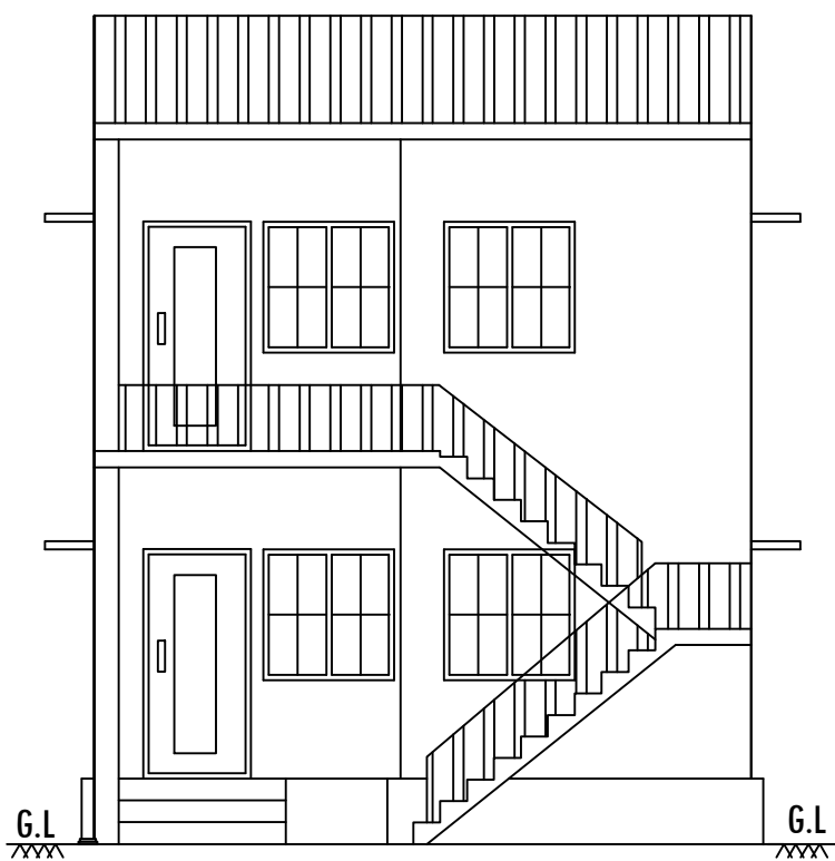
ELEVATION
