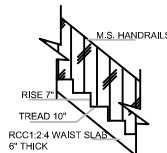
STAIRCASE DETAILS SCALE: 1:20
