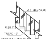
STAIRCASE DETAILS SCALE: 1:20
