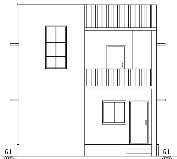
ELEVATION
