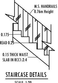
STAIRCASE DETAILS SCALE: 1:20
