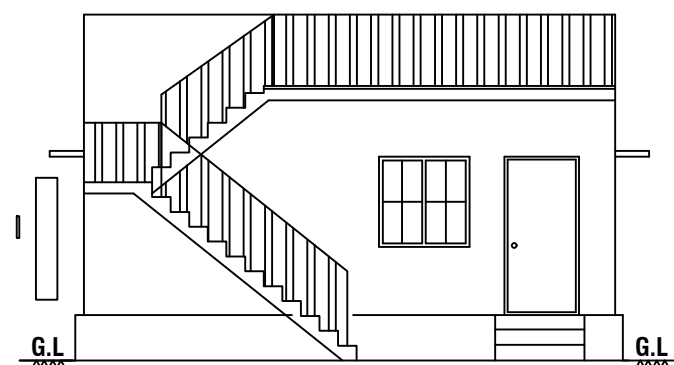
ELEVATION
