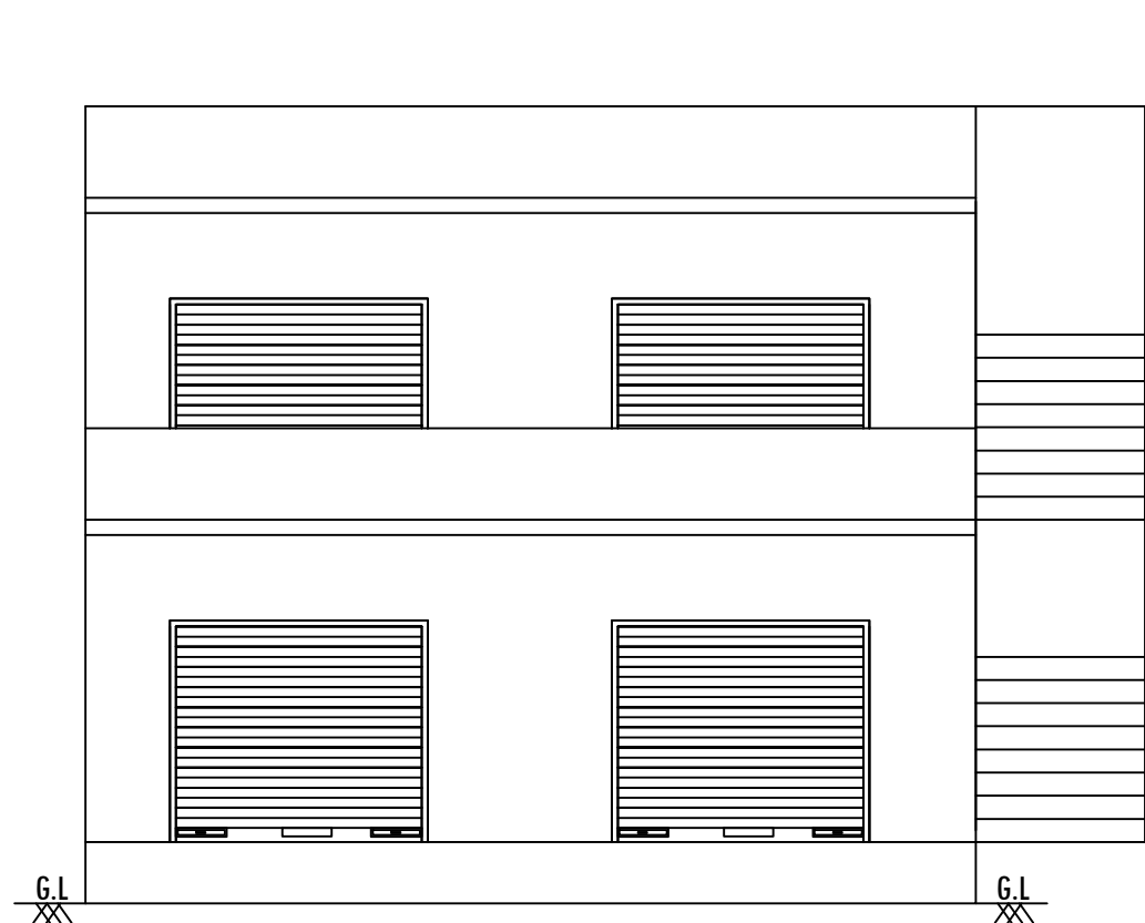
Elevation
