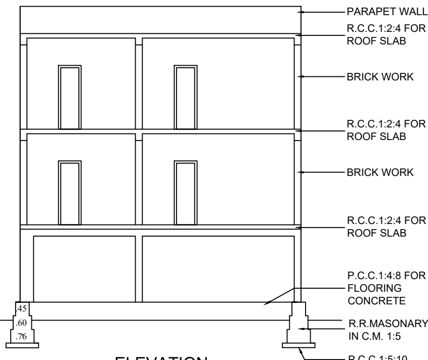
ELEVATION
