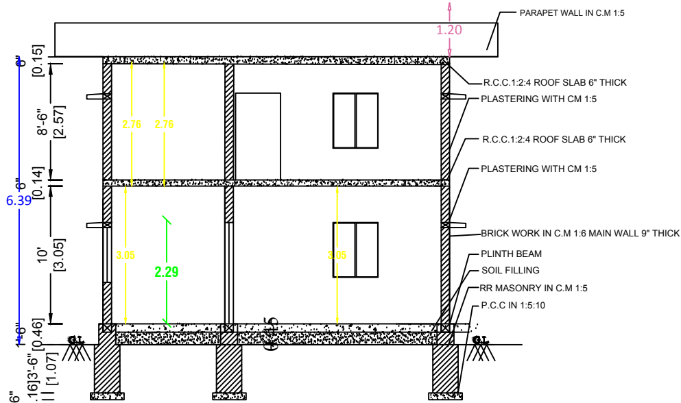
A-B SECTION
