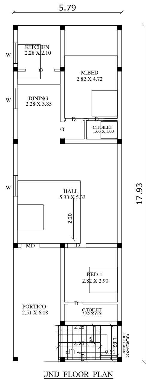
UND FLOOR PLAN
