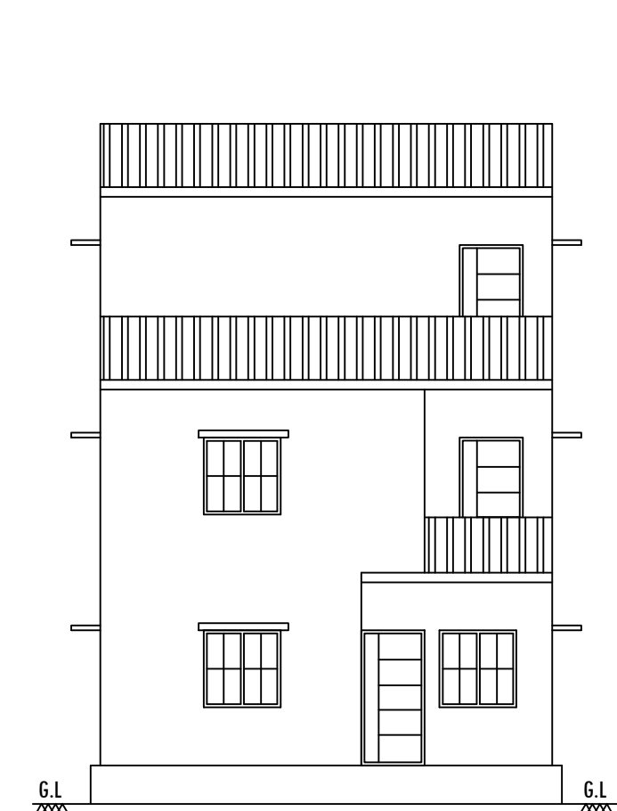
ELEVATION
