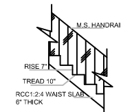
STAIRCASE DETAILS SCALE: 1:20
