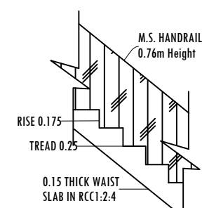
STAIRCASE DETAILS SCALE: 1:20
