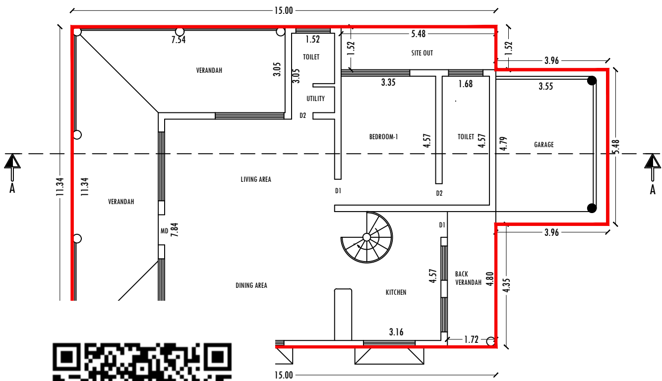
DOOR PLAN
