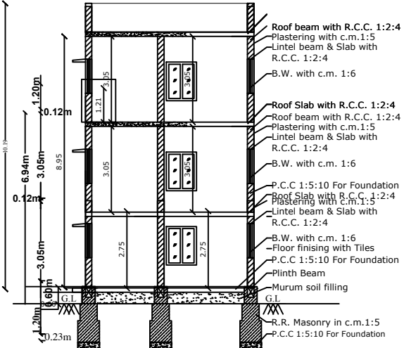
SECTION 'AB'
