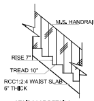
STAIRCASE DETAILS SCALE: 1:20
