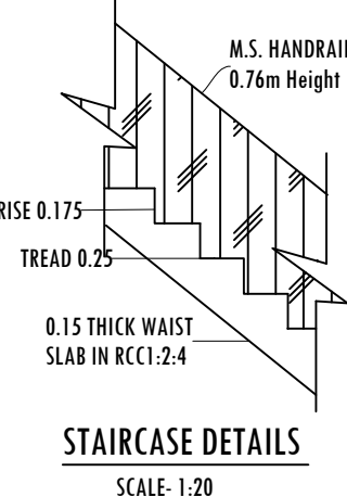
STAIRCASE DETAILS SCALE: 1:20
